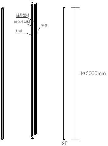
艾瑞-45前立柱 H≤3000mm W=70mm D=25mm
