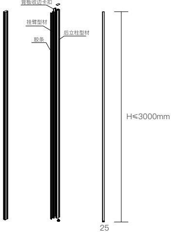
艾瑞-后立柱 H≤3000mm W=45mm D=25mm
