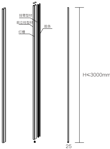
艾瑞-70前立柱 H≤3000mm W=70mm D=25mm
